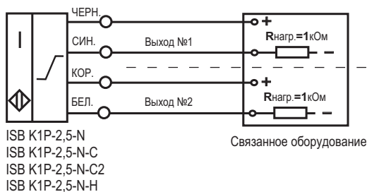
Схема подключения к оборудованию
